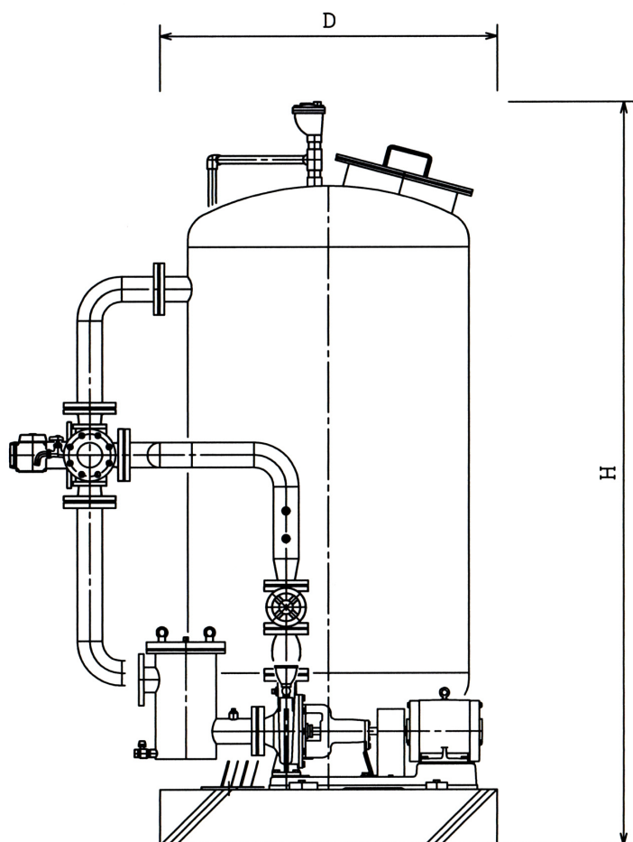
SS製ろ過装置
